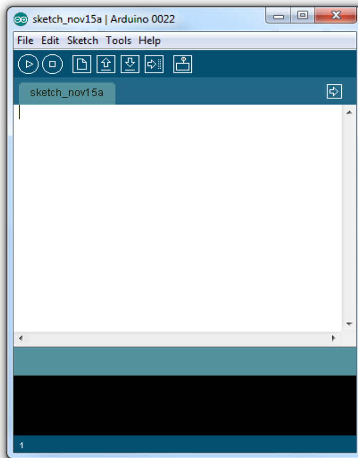
Figure 14. Arduino IDE
